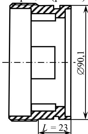
Рисунок 1 – Деталь «Втулка верхняя»
