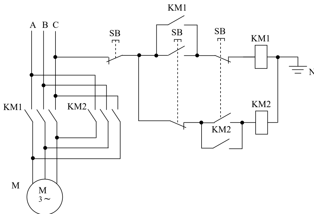
Рисунок 3 – Схема управления реверсивным двигателем с помощью двух магнитных пускателей и трех кнопок
