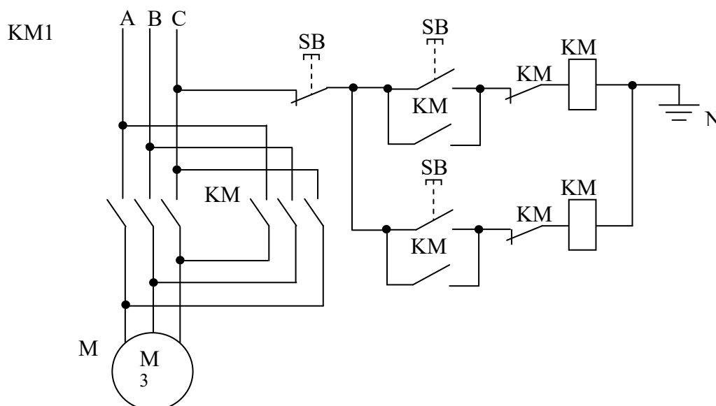
Рисунок 2 – Схема управления реверсивным двигателем с помощью двух магнитных пускателей
