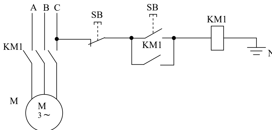
Рисунок 1 – Схема управления двигателем с помощью магнитного пускателя
