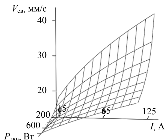
Рисунок 3 - Графическое представление зависимости V_{св} = V_{св}(P, I)
