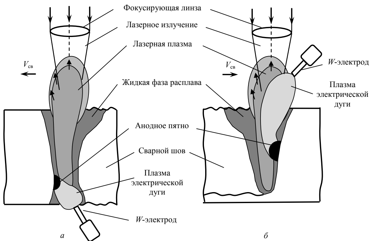
Рисунок 2 - Процесс лазерно-дуговой сварки металлов
